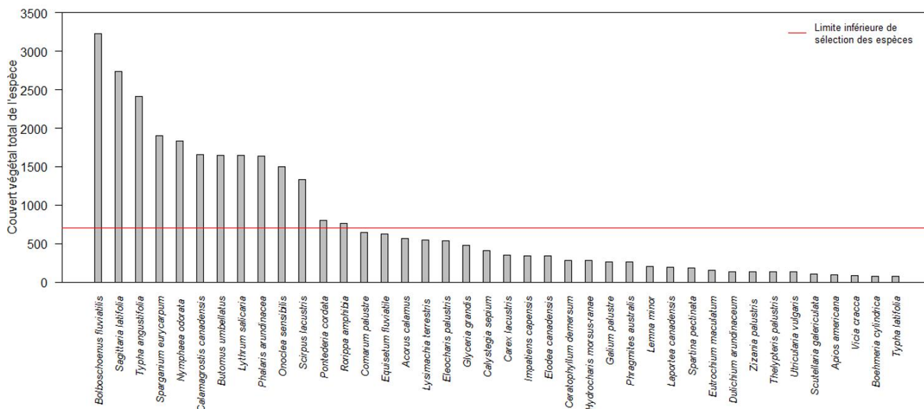
Figure 5: Limite de sélection des espèces végétales selon leur couvert végétal total au lac Saint-Pierre (Québec, Canada) en 2015. Les espèces au-dessus de la limite inférieure de la valeur seuil ont été sélectionnées comme les plus abondantes du lac Saint-Pierre. Cette sélection s'est faite conjointement avec les résultats montrés à la Figure 6.
