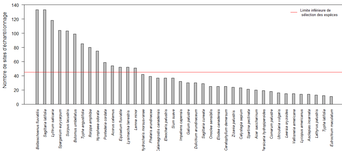
Figure 6 : Limite de sélection des espèces végétales selon le nombre de sites d'échantillonnage où chaque espèce est présente au lac Saint-Pierre (Québec, Canada) en 2015. Les espèces au-dessus de la limite inférieure de la valeur seuil ont été sélectionnées comme les plus abondantes du lac Saint-Pierre. Cette sélection s'est faite conjointement avec les résultats de la Figure 5.
